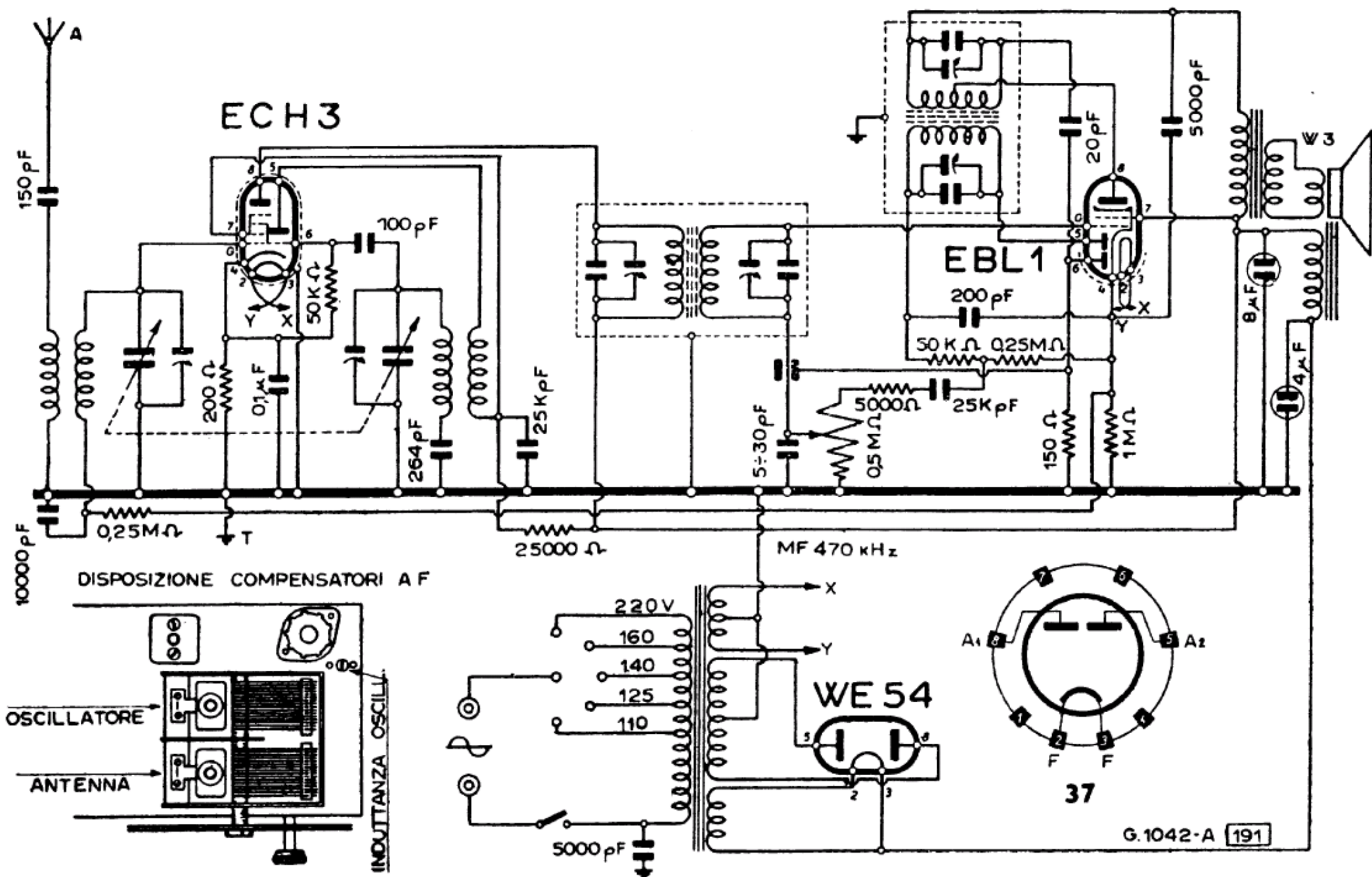
Lo schema elettrico del Phonola 301.
